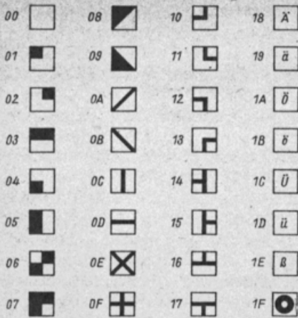
Auf den Adressen 80H...9FH werden die Zeichen von 00H...1FH invers dargestellt.
