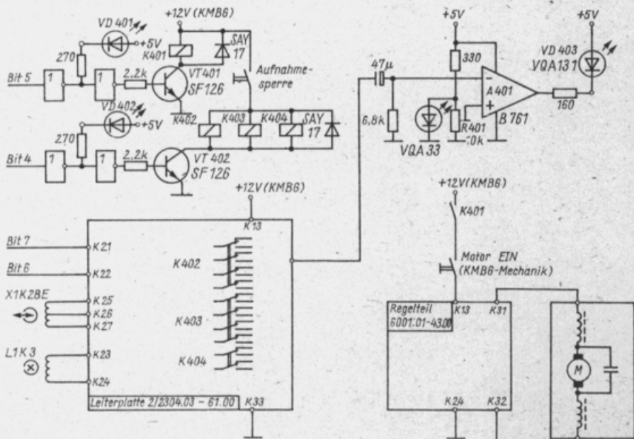
Bild 22: Stromlaufplan der Kassettenmagnetbandgerät-Steuerung
