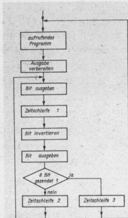
Bild 19: Prinzipieller Ablaufplan einer Byte-Ausgabe
